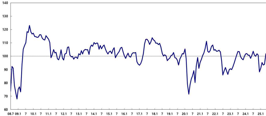
소비자심리지수 1) 추이
