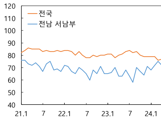
비제조업 인력사정BSI
